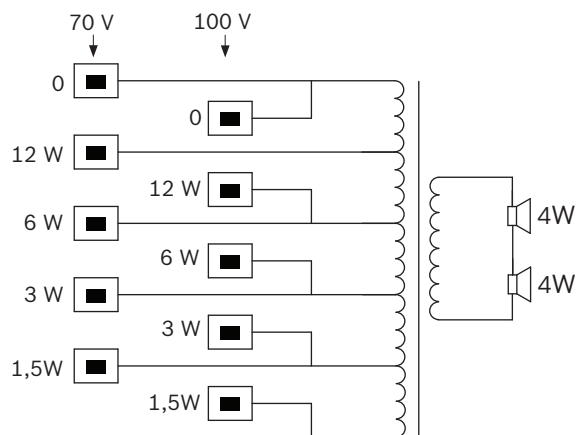
Принципиальная схема
